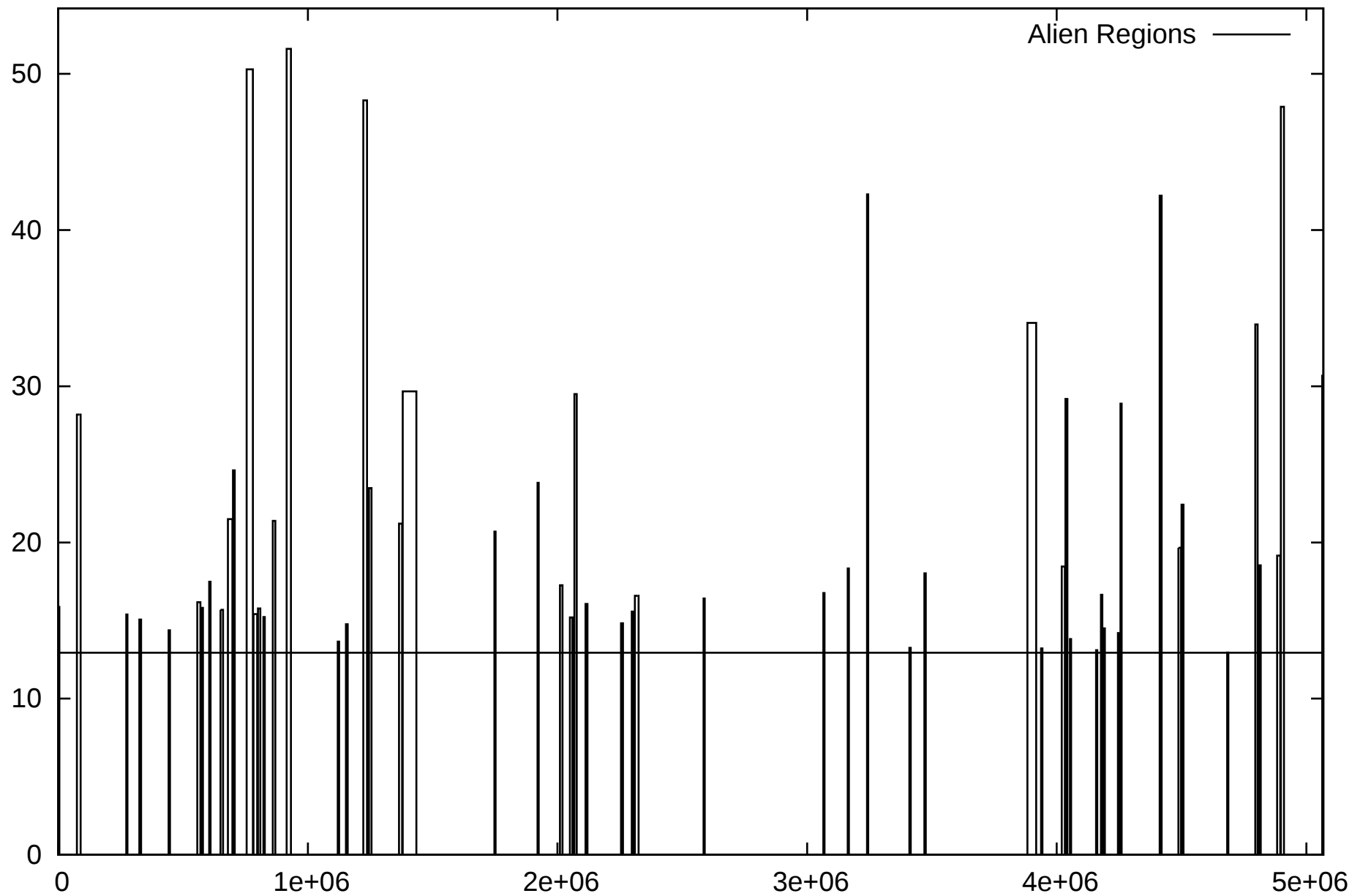
Xarb_juglandis_J303 Alien Regions
